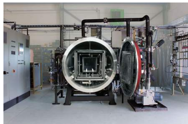
Ofenanlage mit Molybdänheizung und Strahlenschutzblechen aus Molybdän
